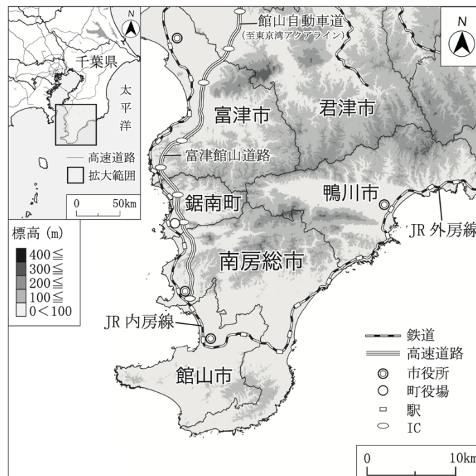
図 1 千葉県南房総地域の概要 IC はインターチェンジの略。 （国土数値情報および基盤地図情報により作成）
