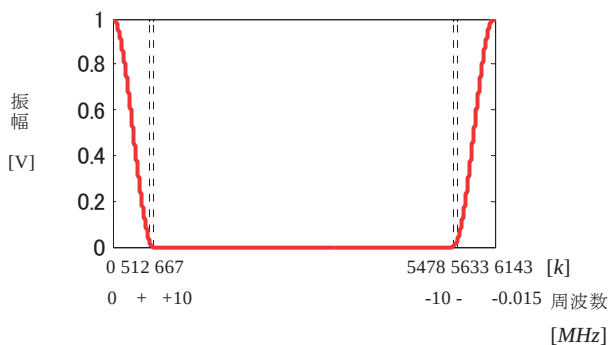
Fig.14 rans er characteristic o raise cosine
