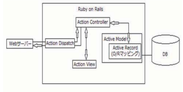
Fig.3 Ruby on Rails の構成
